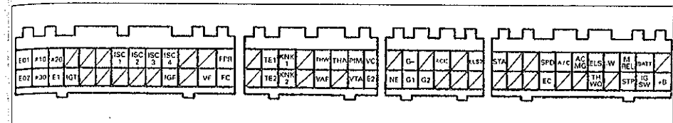
Выводы электронного блока управления (2JZ-GE, JZS155 МКПП).
