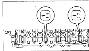
в) Отверните болты крепления крышек №4 и №7.
