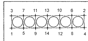
в) Снимите головку блока цилиндров и прокладку.
