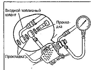
2JZ-GTE.
