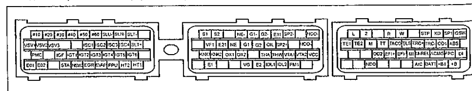
Выводы электронного блока управления (2JZ-GTE, JZA80).
