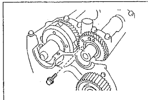
б) Установите распределительный вал, как показано на рисунке.
