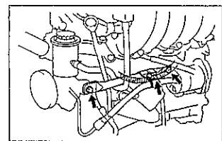
1 - вакуумный шланг, 2 - разъем датчика, 3 - датчик.
