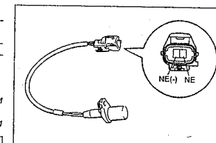
Датчик положения коленчатого вала.
