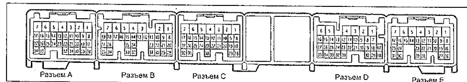
Выводы электронного блока управления (1JZ-FSE, JZX X11#).
