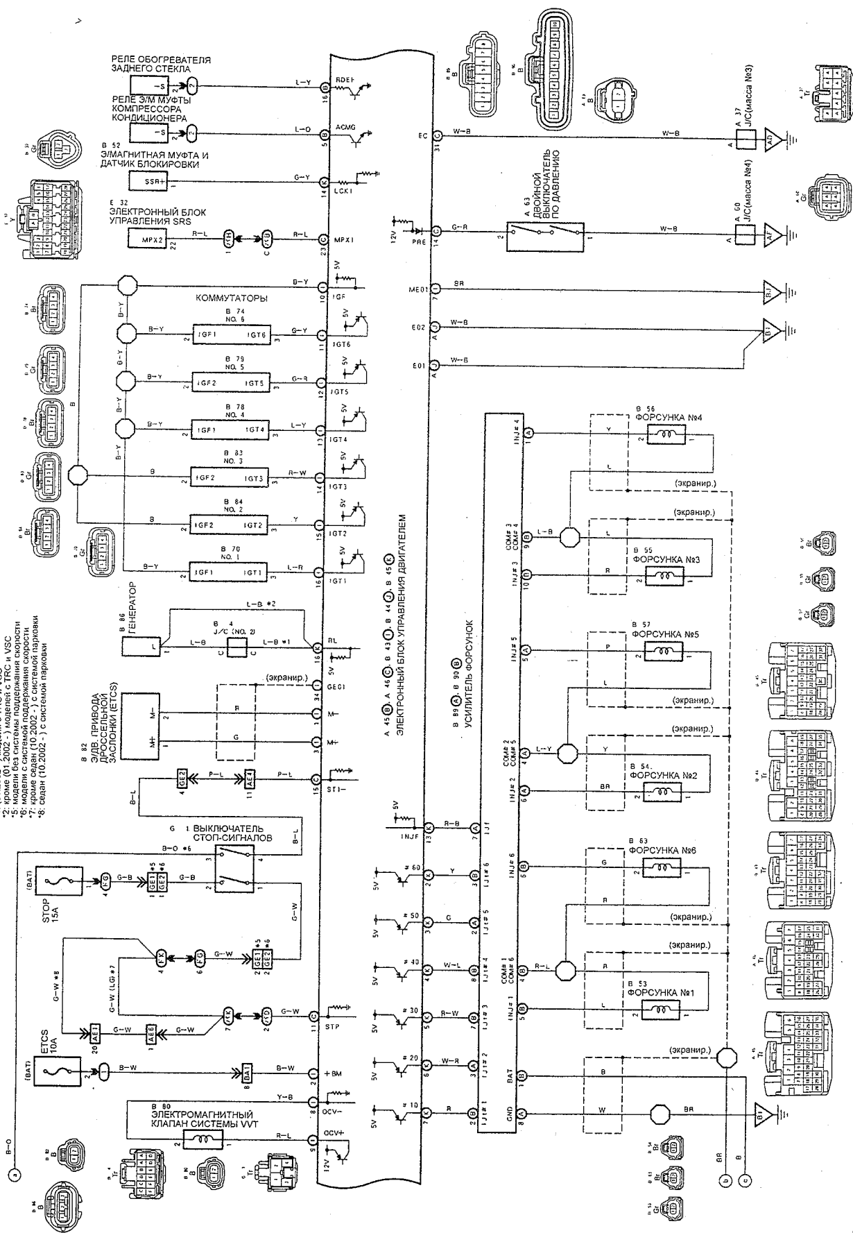
Схема 7 (продолжение) (Mark II X11#).
