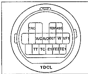
DLC2.
