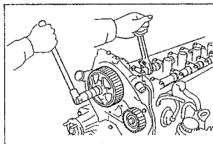
б) Отверните болт крепления шкива.
