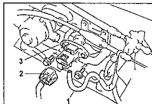
1 - вакуумный шланг, 2 - разъем датчика, 3 - датчик.
