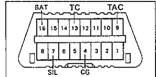
DLC3.
