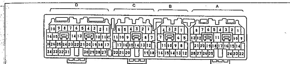
Выходы электронного блока управления (JZS13#, 2JZ-GE, с 10.1991 г.).
