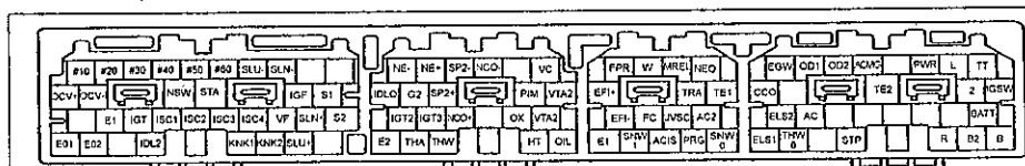
Выходы электронного блока управления (2JZ-GE, JZX100 с 09.1996 г.).
