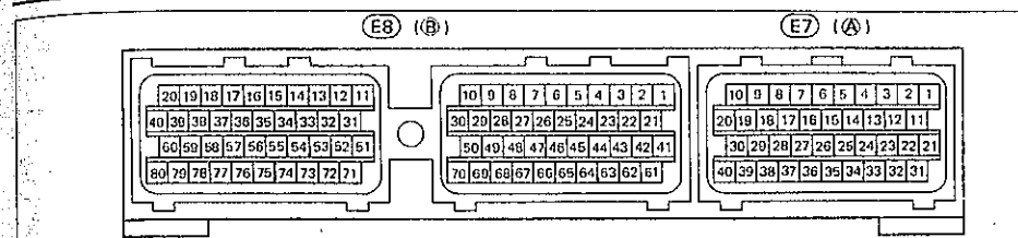
Выводы электронного блока управления (2JZ-GE, JZS14# (GS300) с 1995 г.).
