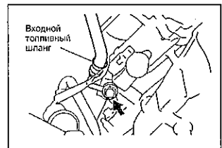
2JZ-GE (JZS155).
