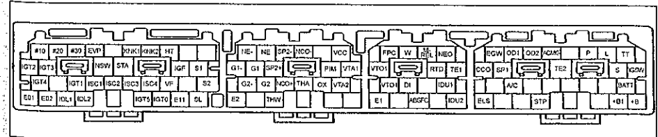
Выводы электронного блока управления (1JZ-GTE, JZX90).
