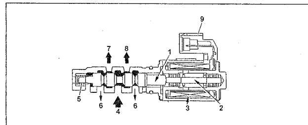
Клапан системы VVT-i (1JZ-GE). 1 - золотник, 2 - плунжер, 3 - обмотка, 4 - масло (напор), 5 - пружина, 6 - масло (на слив), 7 - к поршню (вперед), 8 - к поршню (назад), 9 - разъем.
