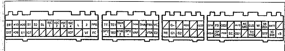
Выводы электронного блока управления (2JZ-GE, JZS155 АКПП).
