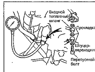
2JZ-GE (JZS165).
