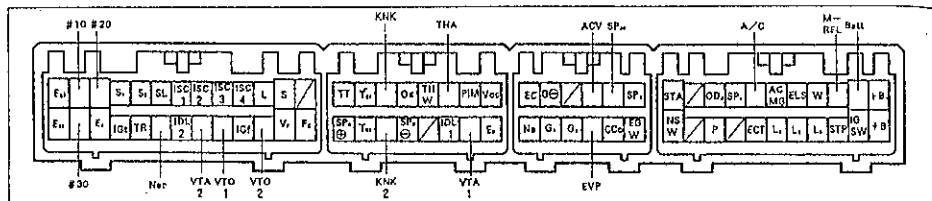
Выходы электронного блока управления (JZS13#, 1JZ-GE, с 10.1991 г.).
