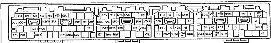
Выходы электронного блока управления (1JZ-GE, JZX100 2WD с 09.1996 г.) (* - тип 1, ** - тип 2).
