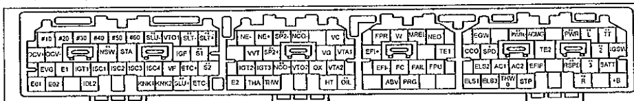
Выходы электронного блока управления (1JZ-GTE, JZX100 с 09.1996 г.) (* - МКПП, ** - АКПП).
