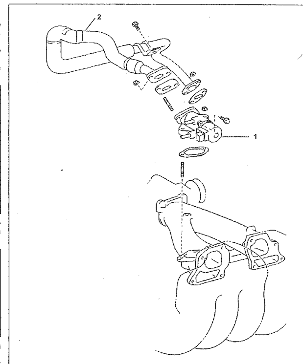
Система EGR (1JZ-FSE). 1 - клапан EGR, 2 - охладитель EGR.
