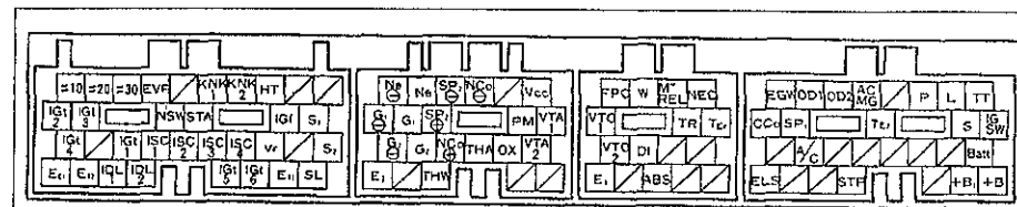
Выходы электронного блока управления (1JZ-GTE, JZZ30).
