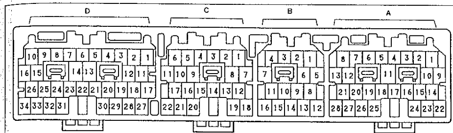
Выводы электронного блока управления (JZS13#, 2JZ-GE, с 08.1993 г.).
