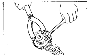
б) Поворачивая спецприспособление вправо, удалите технологический болт из вспомогательной шестерни.
