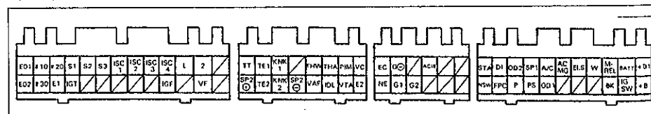
Выводы электронного блока управления (2JZ-GE, JZS133).
