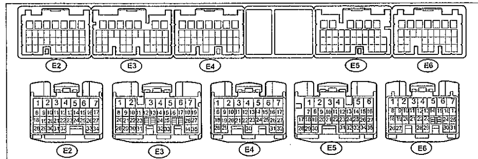
Выводы электронного блока управления (2JZ-GE, JZS16# (GS300) с 2002 г.).
