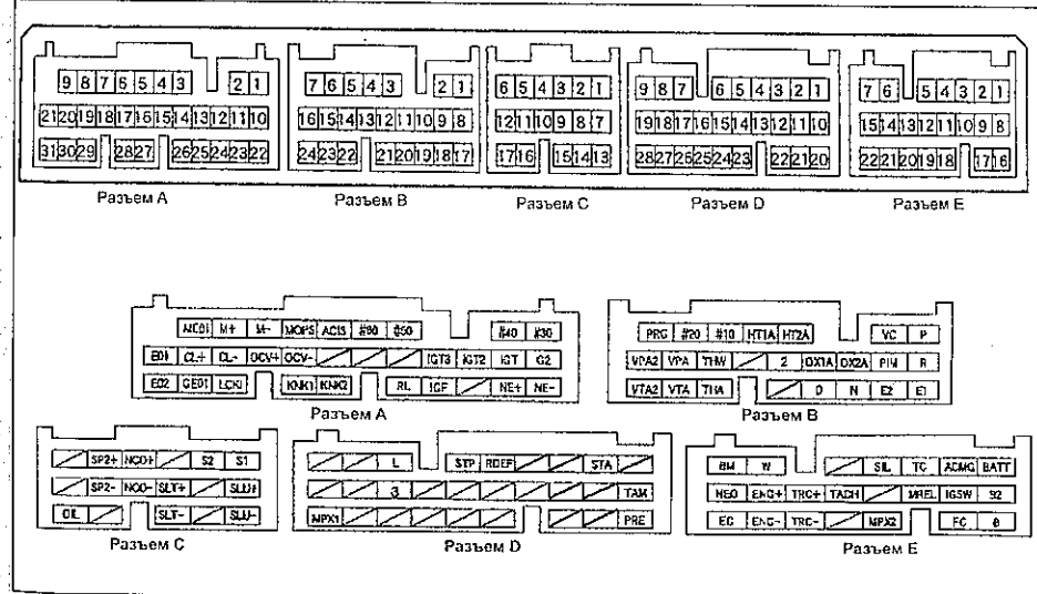
Выводы разъема электронного блока управления (1JZ-GE, Mark II X11# с 2000 г.).
