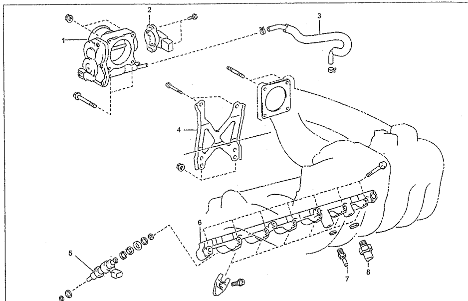
Система впрыска топлива (1JZ-FSE) [1]. 1 - корпус дроссельной заслонки, 2 - датчик положения дроссельной заслонки, 3 - шланг №5 перепуска охлаждающей жидкости, 4 - кронштейн корпуса дроссельной заслонки, 5 - форсунка, 6 - топливный коллектор (рампа), 7 - перепускной клапан, 8 - датчик давления топлива.
