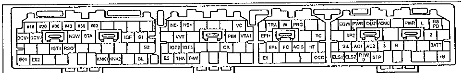
Выходы электронного блока управления (1JZ-GE, JZX105 4WD с 09.1996 г.) (* - тип 1, ** - тип 2).
