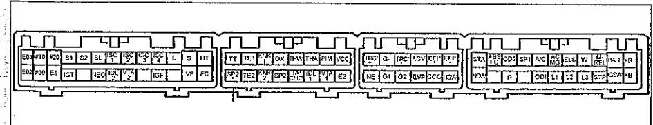
Выводы электронного блока управления (1JZ-GE, JZX90).
