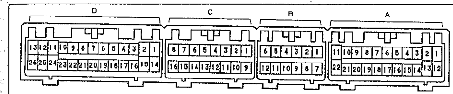
Выводы электронного блока управления (JZS13#, 1JZ-GE, с 08.1993 г.).
