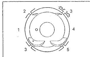
2JZ-GE VVT-i. 1 - метка "перед", 2 - верхний скребок масляного кольца, 3 - верхнее компрессионное кольцо, 4 - расширитель масляного кольца, 5 - нижний скребок масляного кольца, 6 - нижнее компрессионное кольцо.
