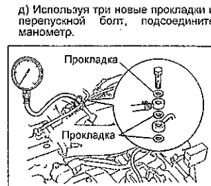
2JZ-GE (JZS133).
