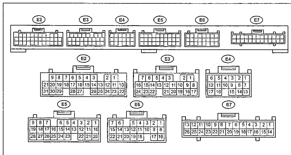
Выводы электронного блока управления (2JZ-GE, JZS16# (GS300) с 1998 г.).
