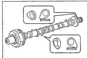
в) Отверните болты крепления крышек подшипников в следующем порядке: №2 - №6 - №4 - №5.
