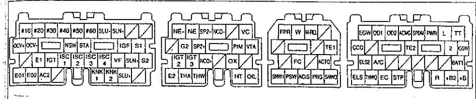
Выводы электронного блока управления (2JZ-GE, JZS155 VVT-i).
