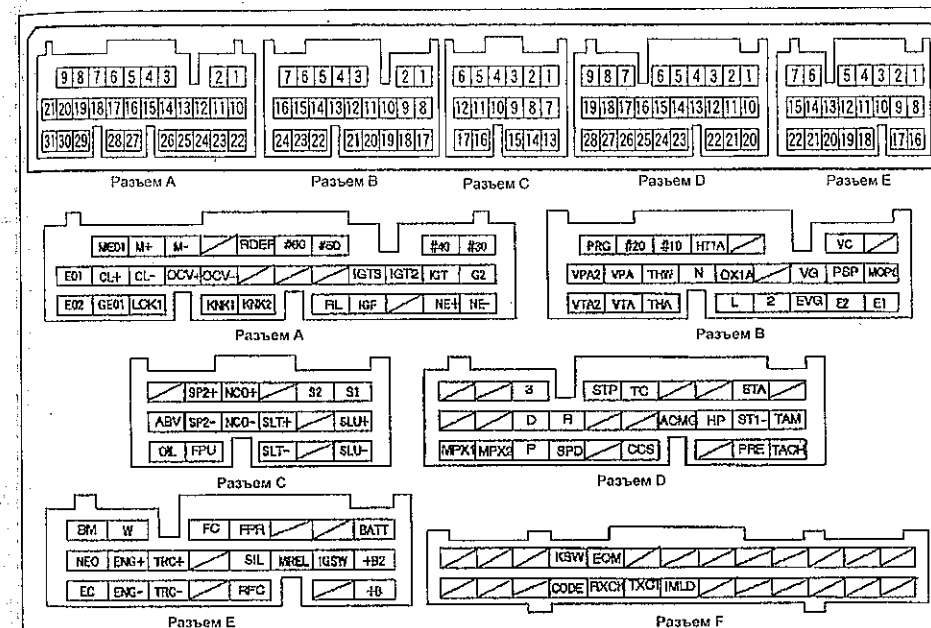
Выводы разъема электронного блока управления (1JZ-GTE, Mark II X11# с 2000 г.).
