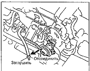
2JZ-GTE.
