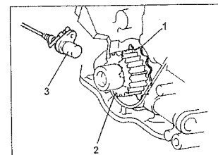
Датчик положения коленчатого вала. 1 - ротор, 2 - шкив коленчатого вала, 3 - датчик.
