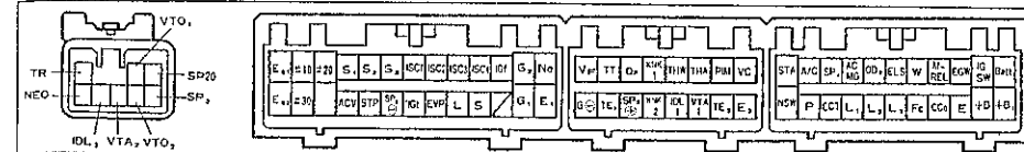
Выходы электронного блока управления (JZS13#, 1JZ-GE, с 08.1990 г.).
