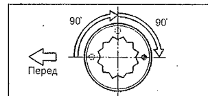
д) Нанесите метки краской на переднюю часть болтов головки блока цилиндров.
