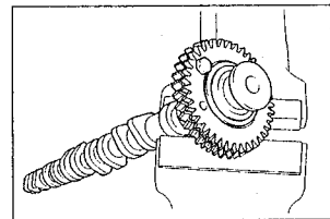
б) Поворачивая спецприспособление вправо, удалите технологический болт из вспомогательной шестерни.
