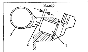
Датчик положения распределительного вала. 1 - датчик, 2 - ротор, 3 - распределительный вал впускных клапанов.
