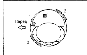
1JZ-FSE. 1 - метка "перед", 2 - нижнее компрессионное кольцо, 3 - верхнее компрессионное кольцо, 4 - масляное кольцо.
